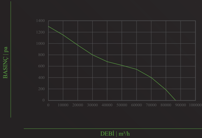
TİFA-PF- 1120-A
