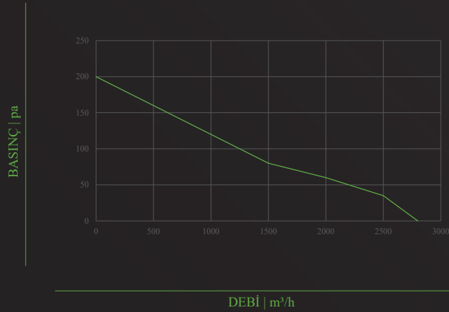
TİFA-PF- 400
