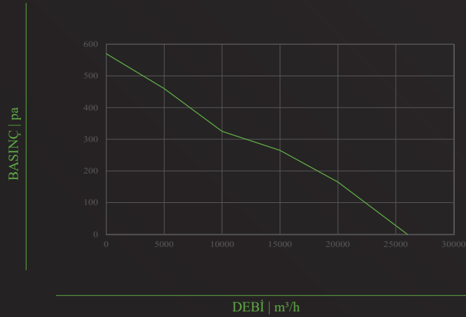
TİFA-PF- 800-A
