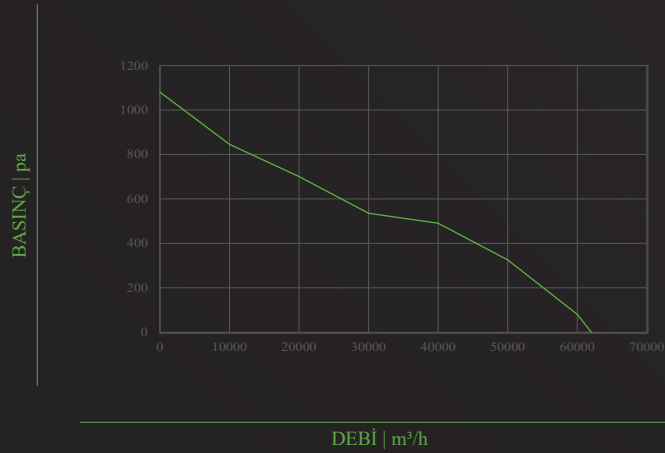
TİFA-PF- 1000-B
