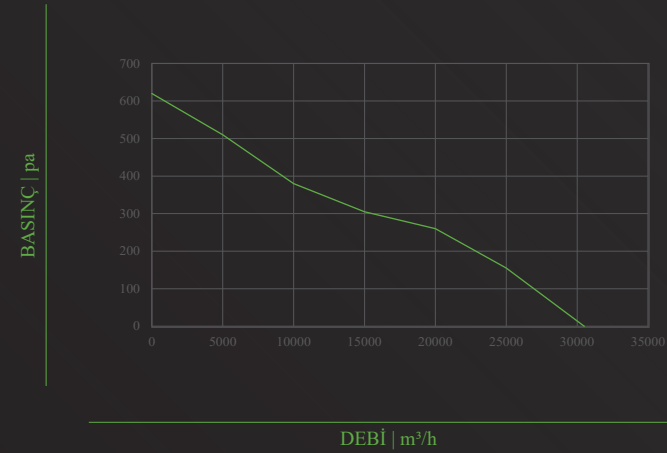
TİFA-PF- 800-B
