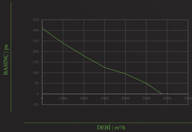
TİFA-PF- 500
