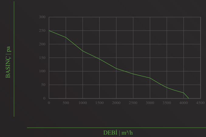
TİFA-PF- 450
