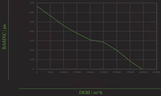
TİFA-PF- 900-A
