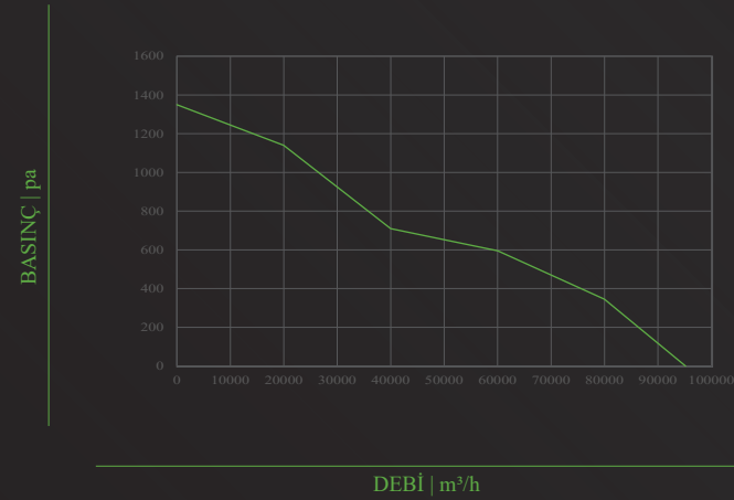
TİFA-PF- 1120-B
