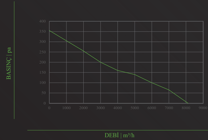
TİFA-PF- 560
