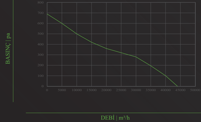
TİFA-PF- 900-B
