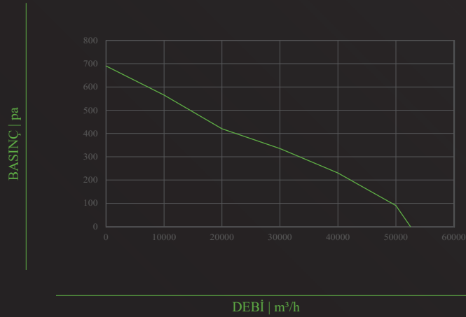
TİFA-PF- 1000-A
