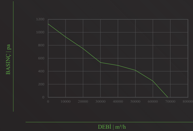
TİFA-PF- 1000-C
