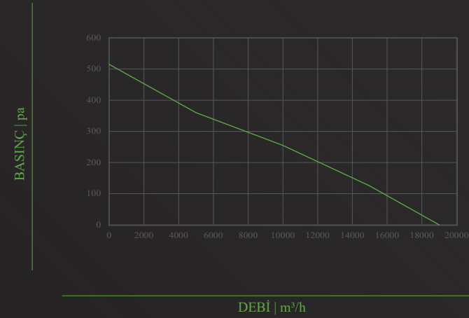
TİFA-PF- 710
