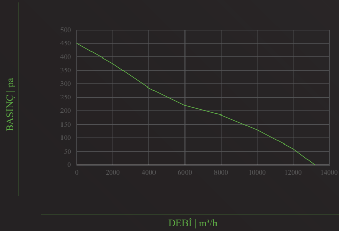
TİFA-PF- 630
