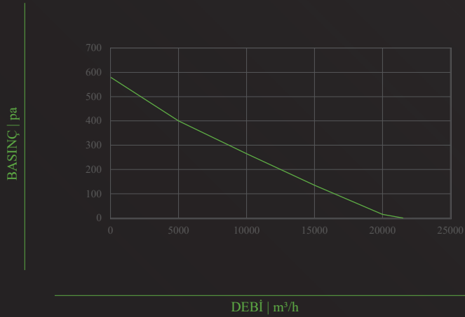
TİFA-VAF-800-A
