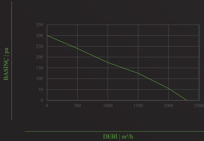
TİFA-VAF-500
