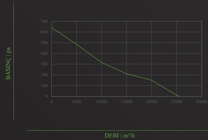
TİFA-VAF-800-B
