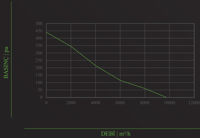
TİFA-VAF-630
