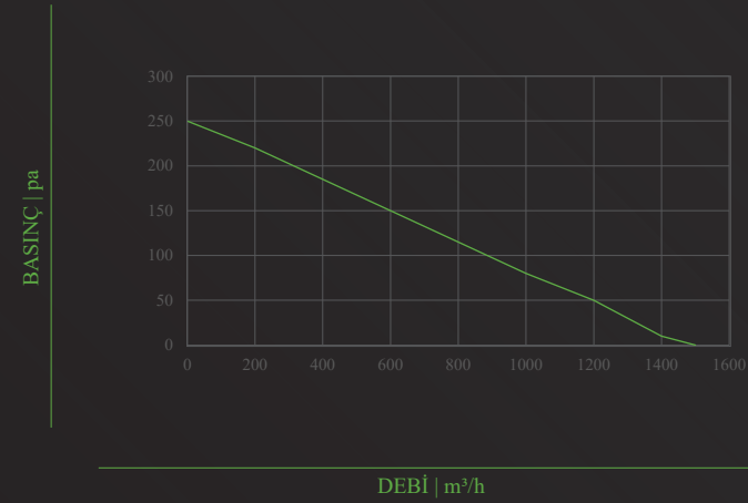
TİFA-VAF-450
