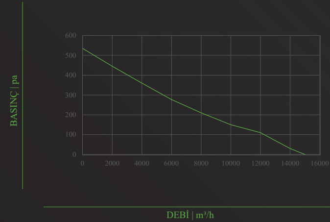
TİFA-VAF-710
