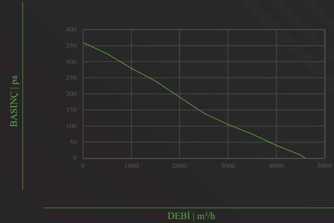
TİFA-VAF-560
